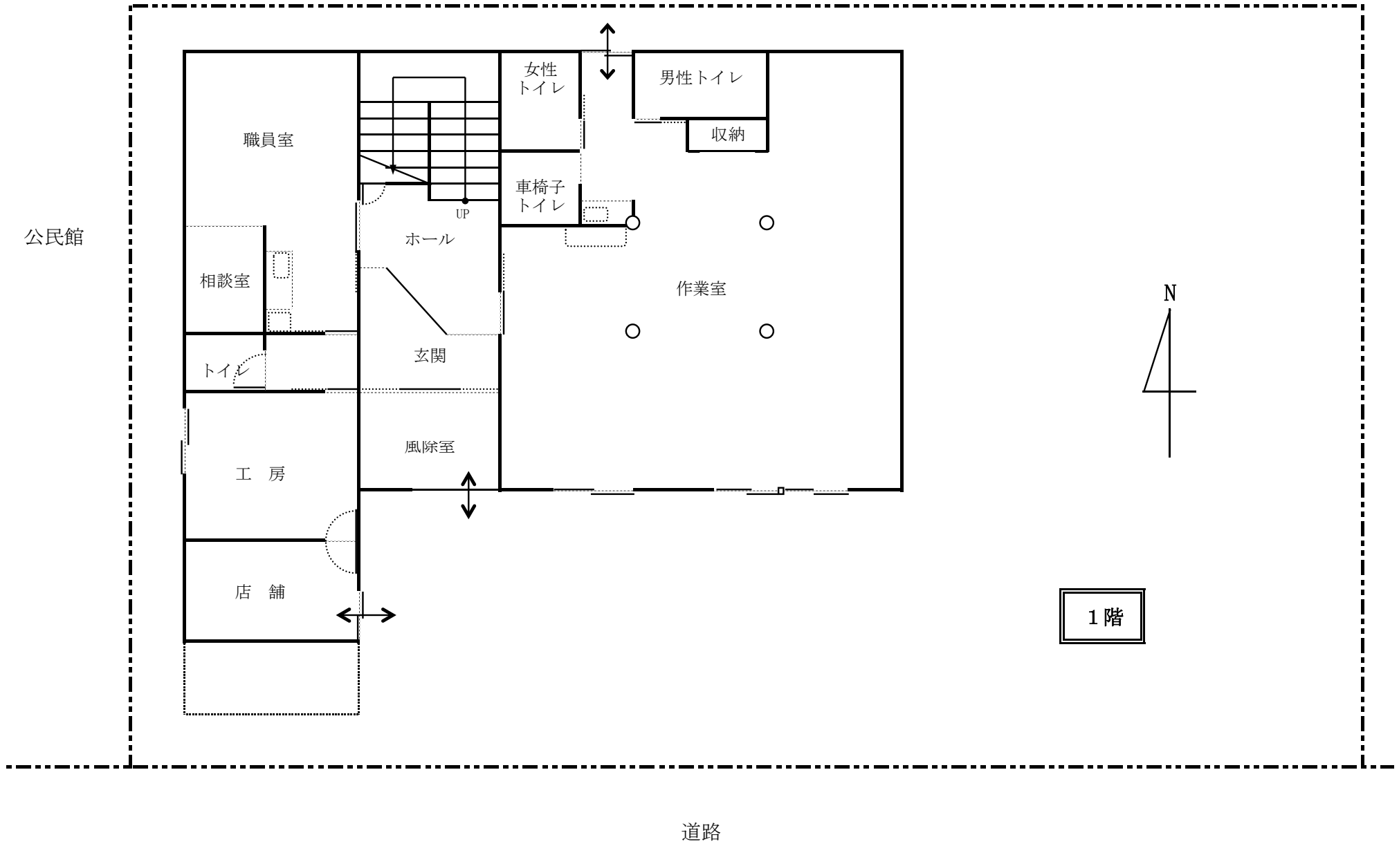
つばさの郷 1階平面図
